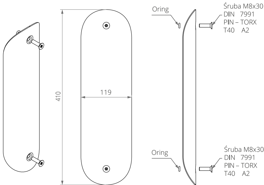
RYSUNEK TECHNICZNY
