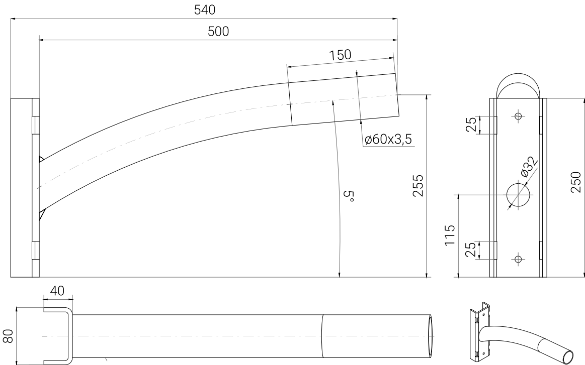
RYSUNEK TECHNICZNY
