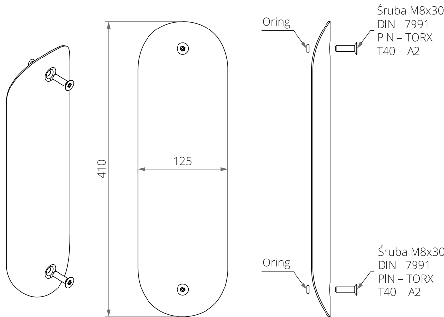
RYSUNEK TECHNICZNY
