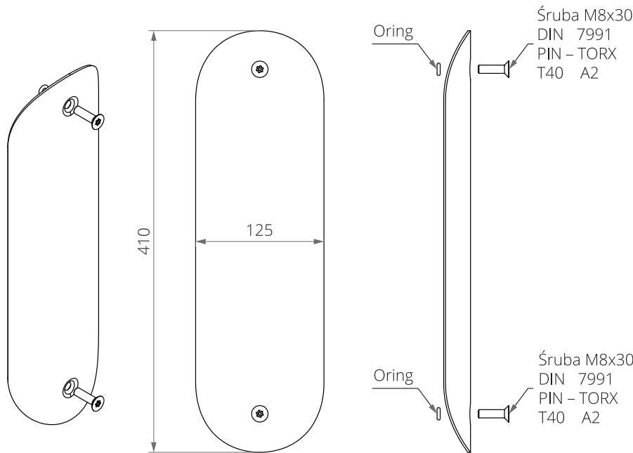
RYSUNEK TECHNICZNY
